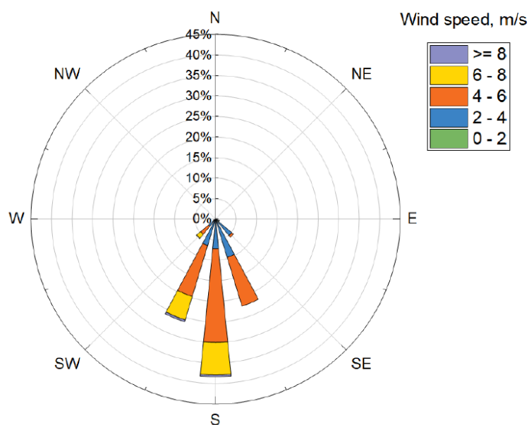
2 paveikslas. Vėjo greitis ir kryptys
